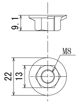
皿ばねナット詳細図
