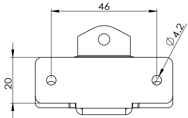
矢视图 A-A
